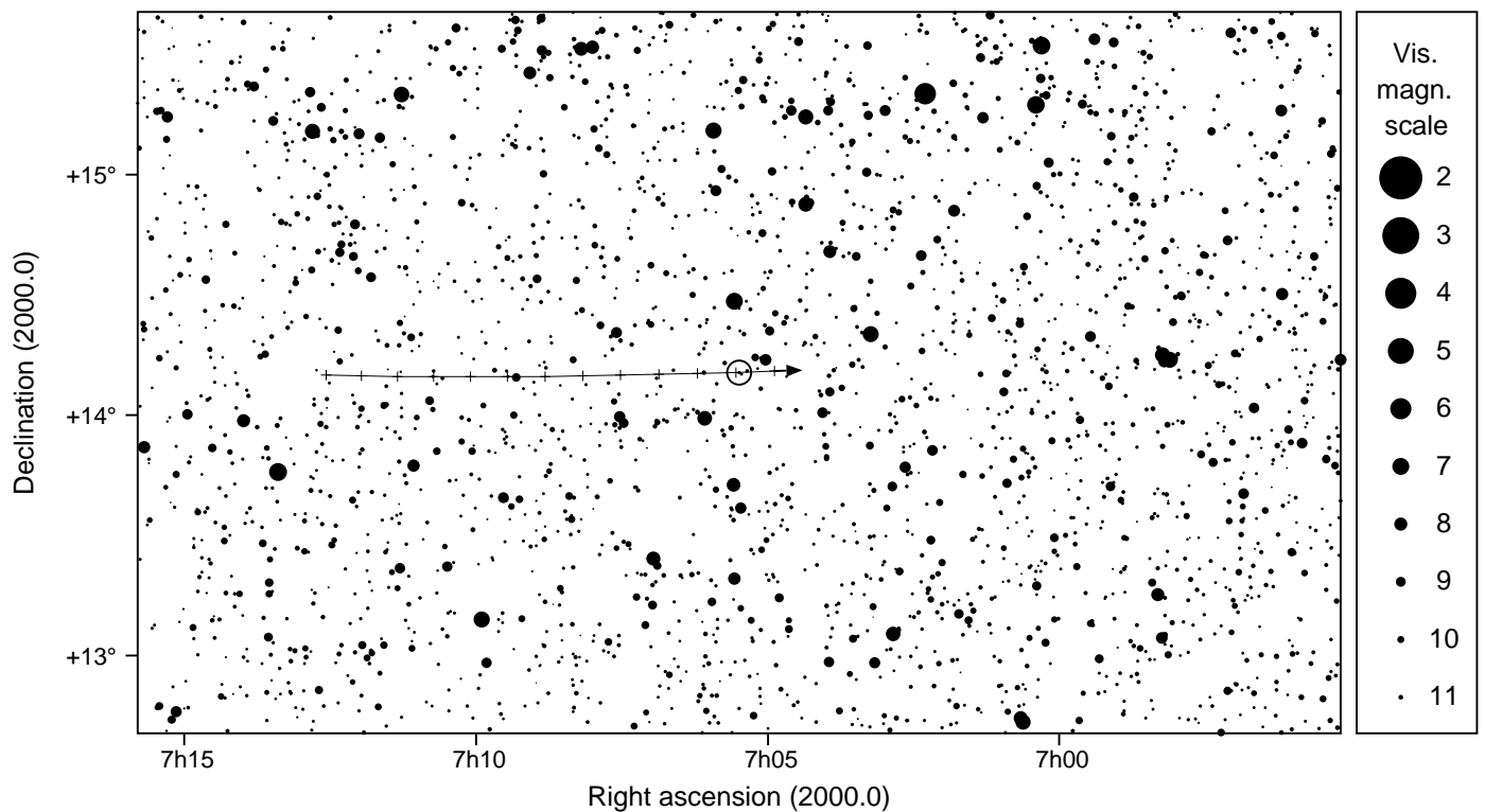
1h52m00s – 2h03m00s; int. 1m
