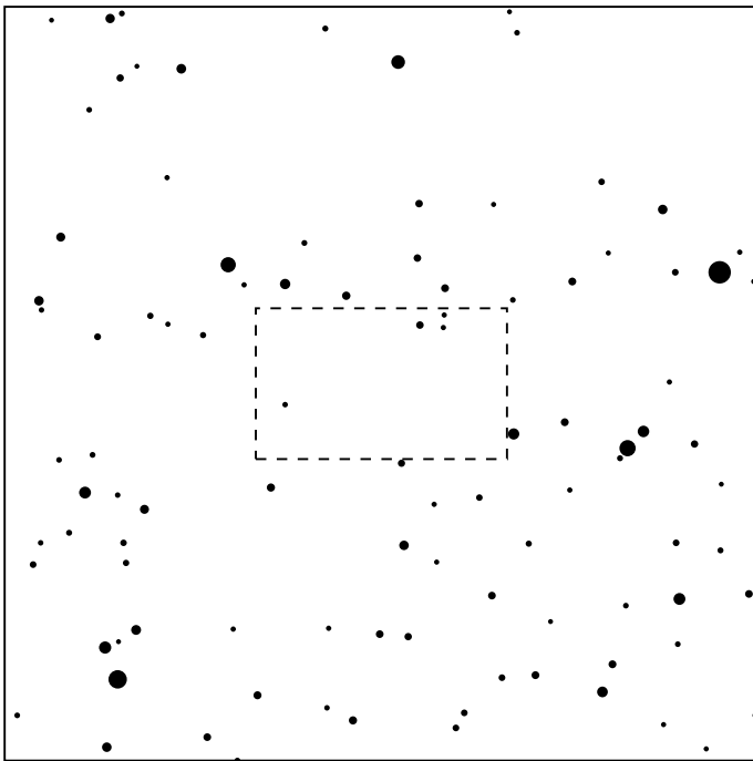
1h52m00s – 2h03m00s; int. 1m
